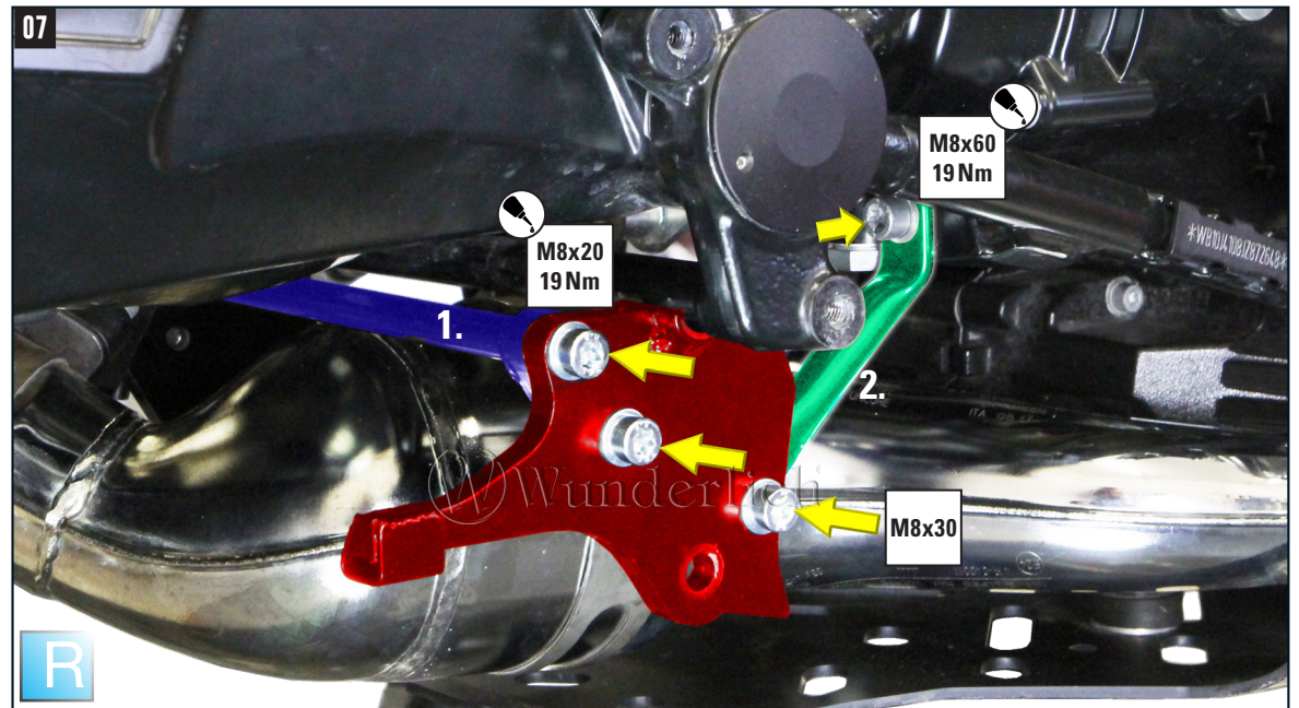
1. Rechten Halter mit der Querstrebe verschrauben. 2. Verdrehsicherung vornontieren und später fest verschrauben! 1. Bolt the right bracket to the cross brace. 2. Pre-assemble the rotation lock and tighten it later on!
