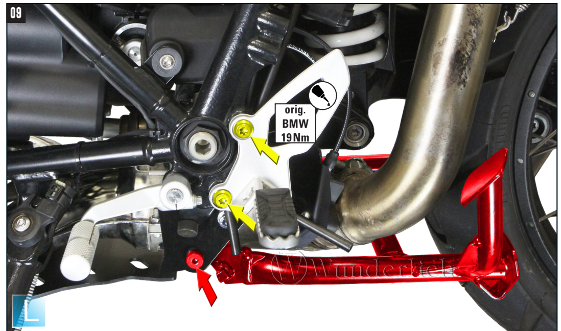
1. Rastenträger montieren 2. Hauptständer lose vormontieren! 1. Mount the footrest support. 2. Loosely pre-assemble the centre stand!
