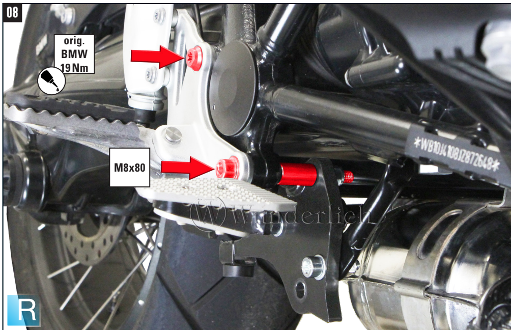
Hülse / spacer D=13,5/ d=8,5/ h= 25,0mm Je nach Modell muss eine der beiden Hülsen verwendet werden. Hülse / spacer D=13,5/ d=8,5/ h= 27,0mm Depending on the model, use one of the sleeves.
